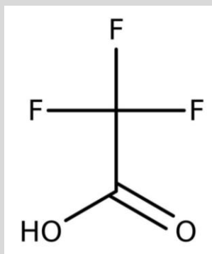
Struktur der Trifluoressigsäure (TFA).
